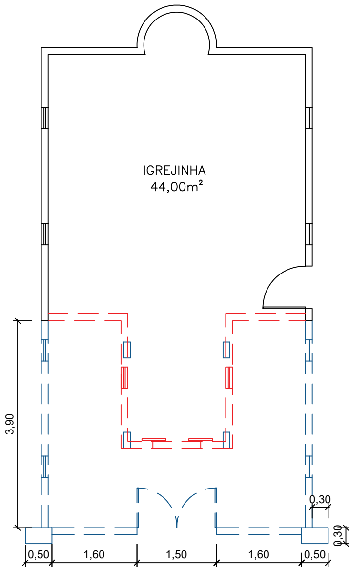
○ PLANTA DE DEMOLIÇÃO E CONSTRUÇÃO 1/75
