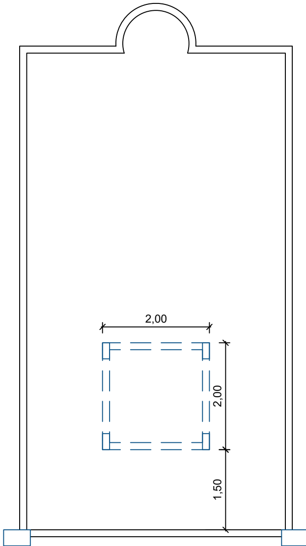
○ PLANTA DE DEMOLIÇÃO E CONSTRUÇÃO – TORRE 1/75
