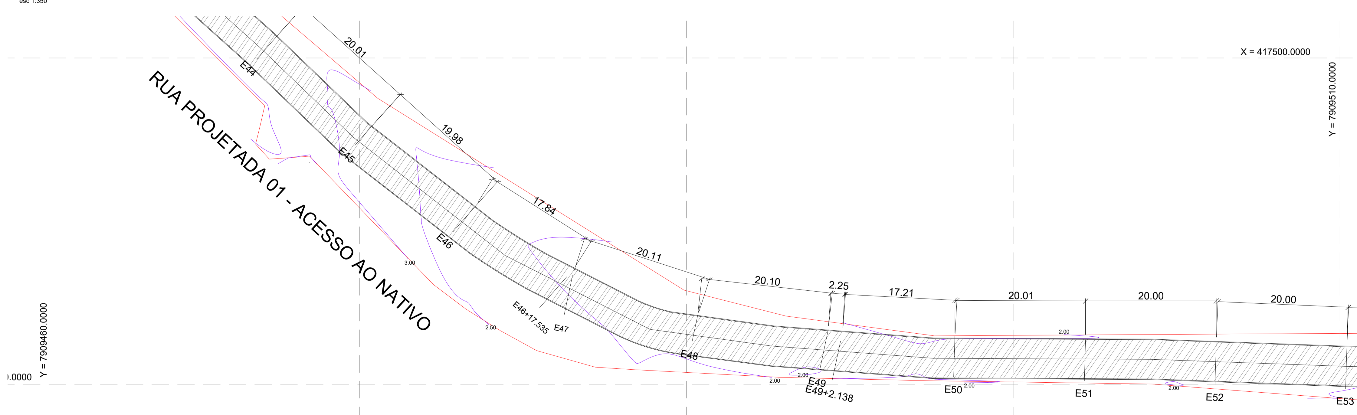
PLANTA BAIXA - PAVIMENTAÇÃO 06 TRECHO 06 esc 1:350
