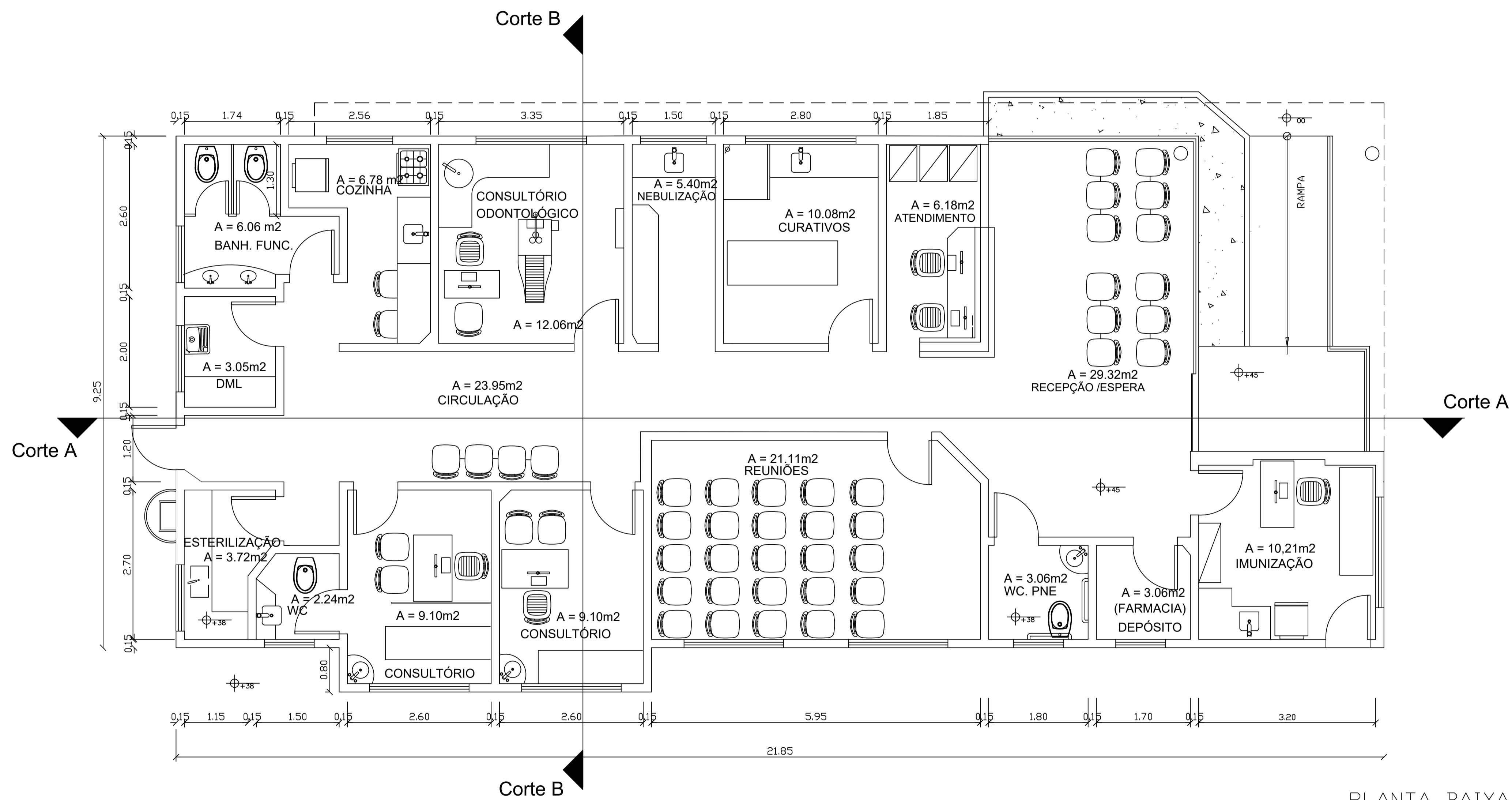
PLANTA BAIXA ESC. 1/50
