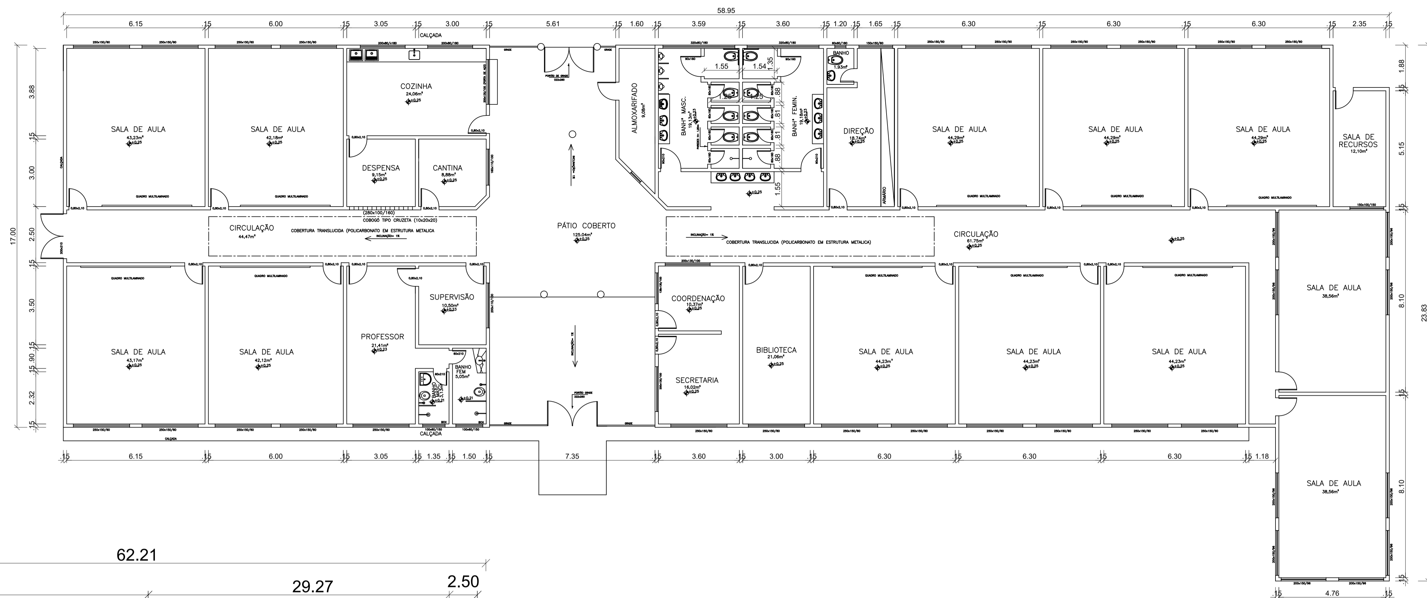
LEVANTAMENTO ESC.-----1/100
