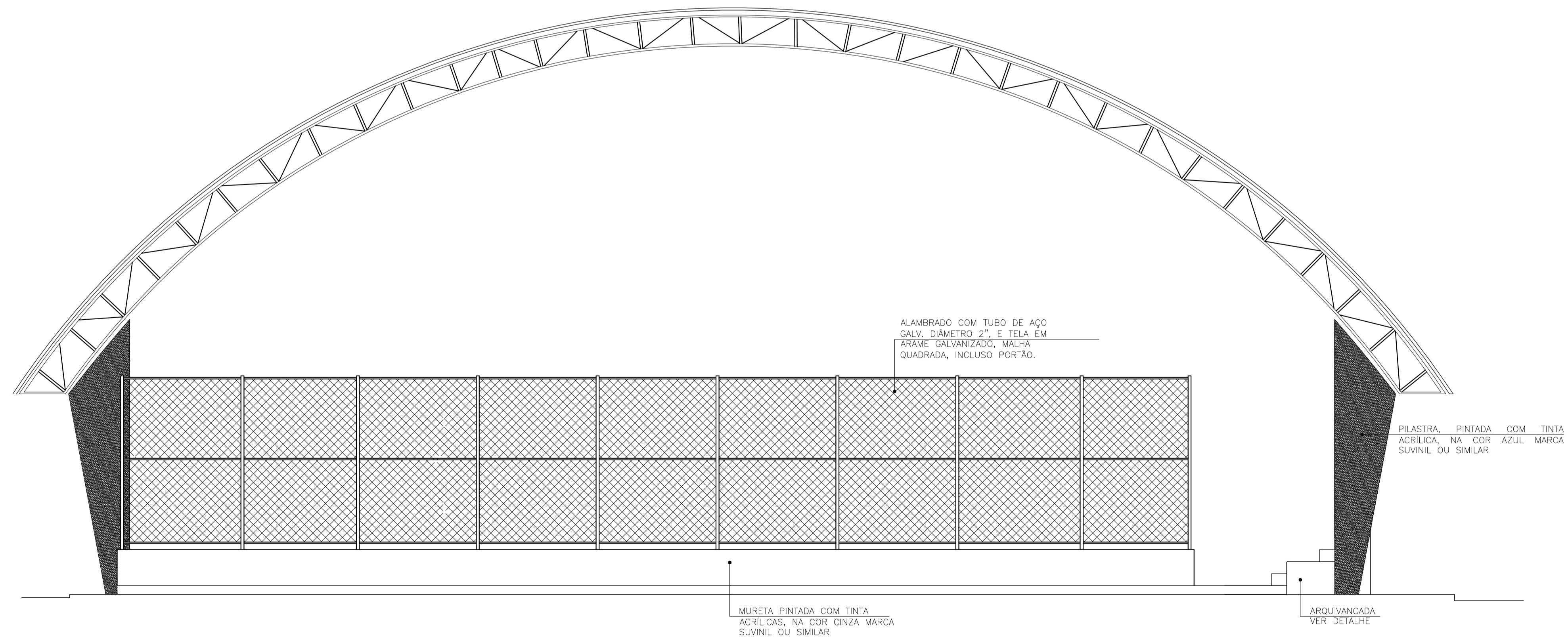
FACHADA 2 ESC: 1/50
