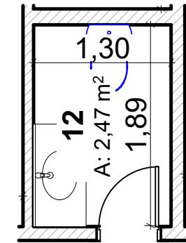
DETALHE 12 1:50
