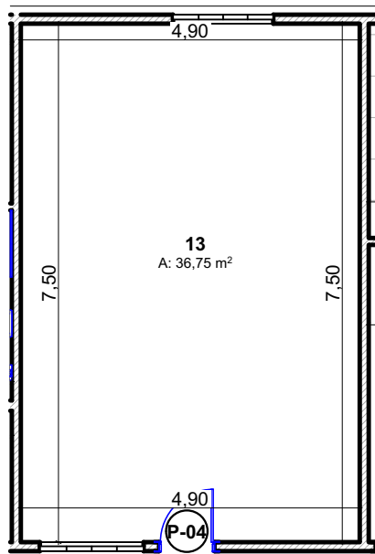
DETALHE 13
