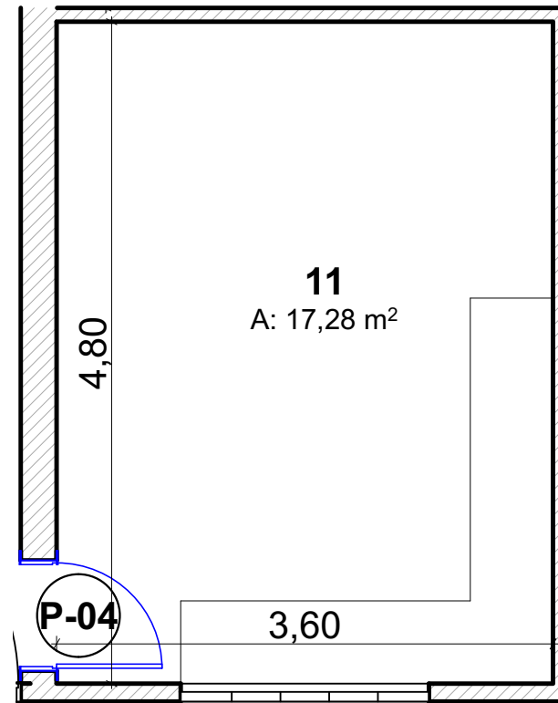
DETALHE 11 1:50
