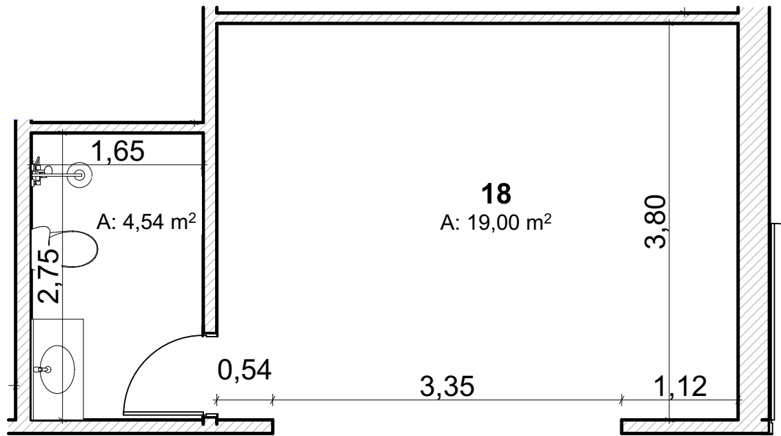
DETALHE 18
