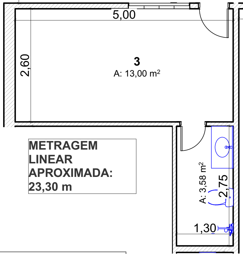
DETALHE 03 1:50
