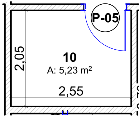
DETALHE 10 1:50
