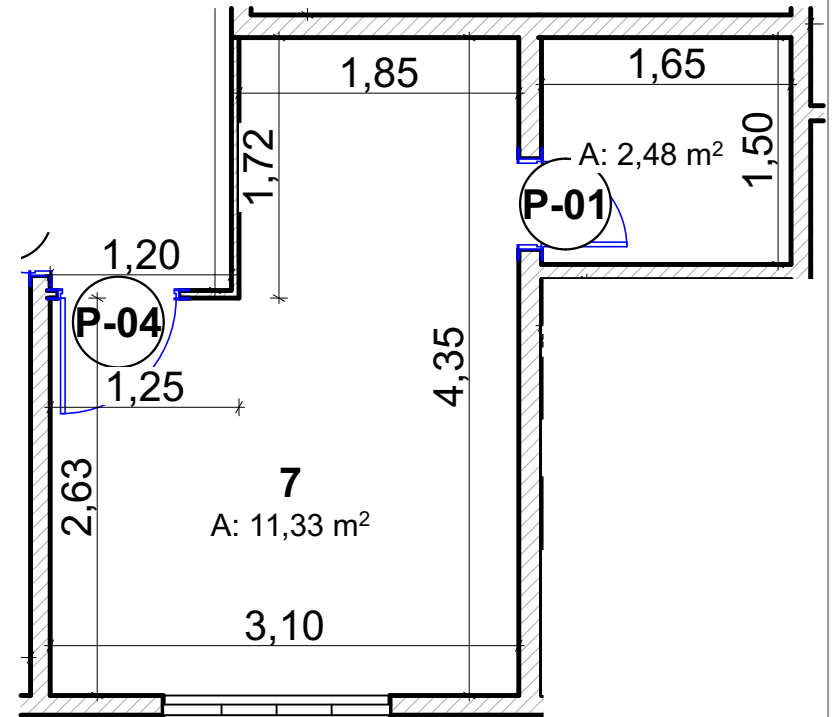
DETALHE 07
