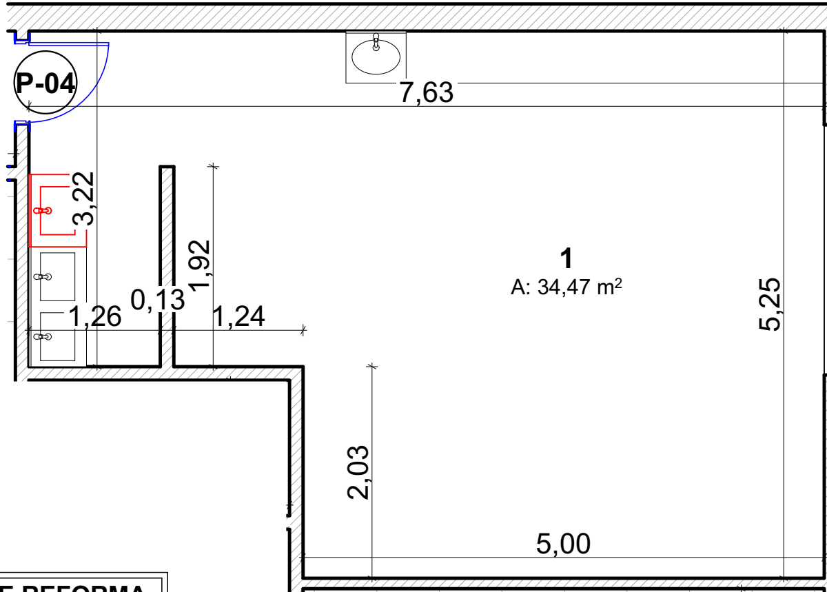
DETALHE 01 1:50
