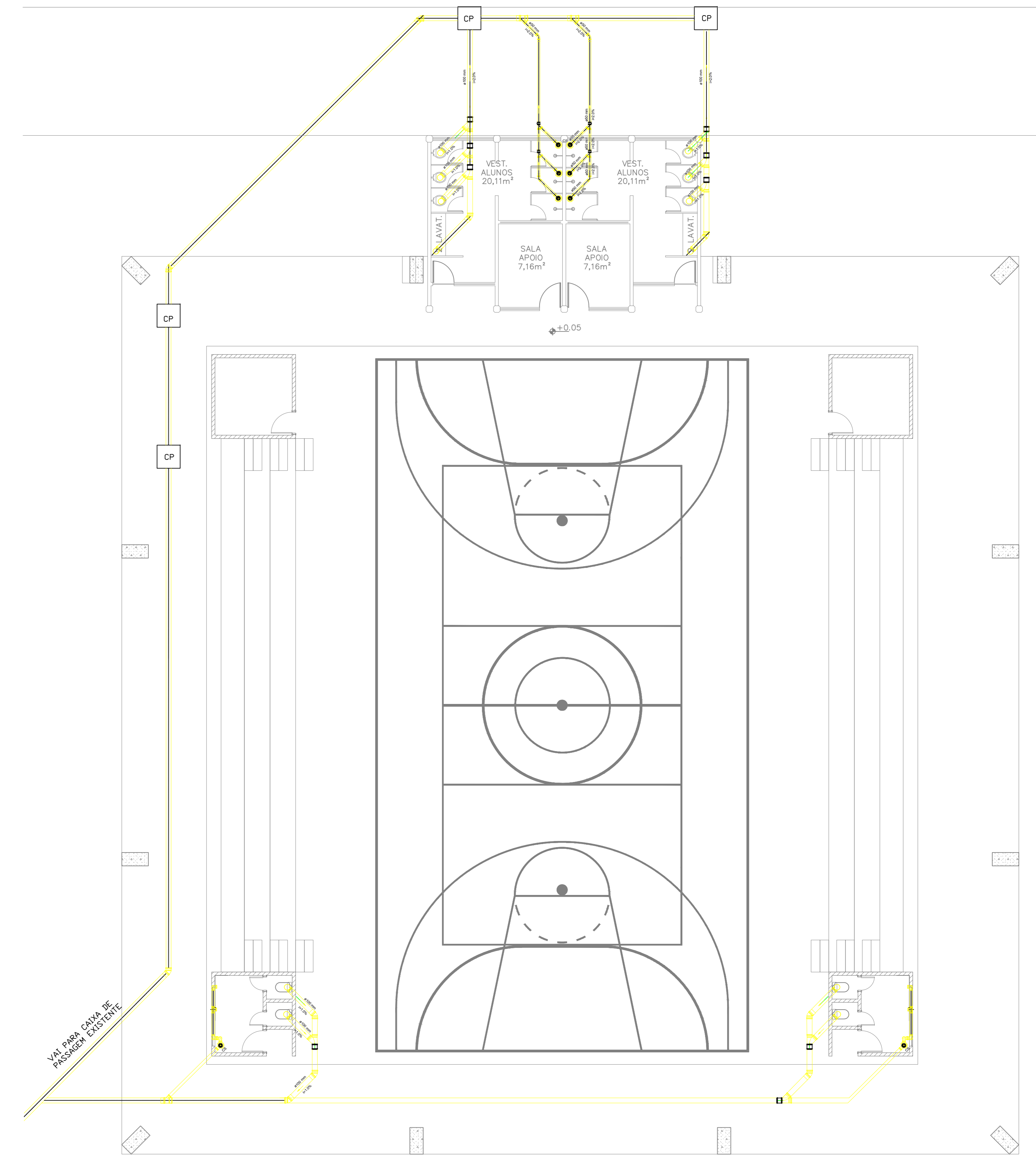
HIDROSSANITÁRIO DA QUADRA ESC. 1/100
