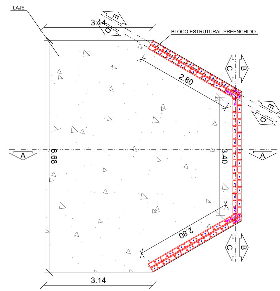
SEÇÃO TIPO LAJE-(ENTRADA) SEM ESCALA
