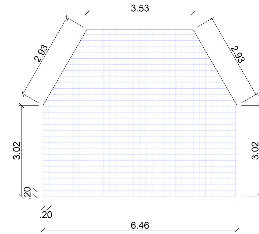
PLANTA BAIXA DE FORMA DA LAJE SEM ESCALA
