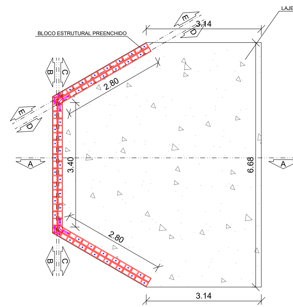
SEÇÃO TIPO LAJE-(SAÍDA) SEM ESCALA
