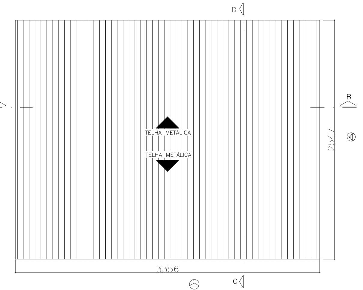
COBERTURA ESC: 1/250
