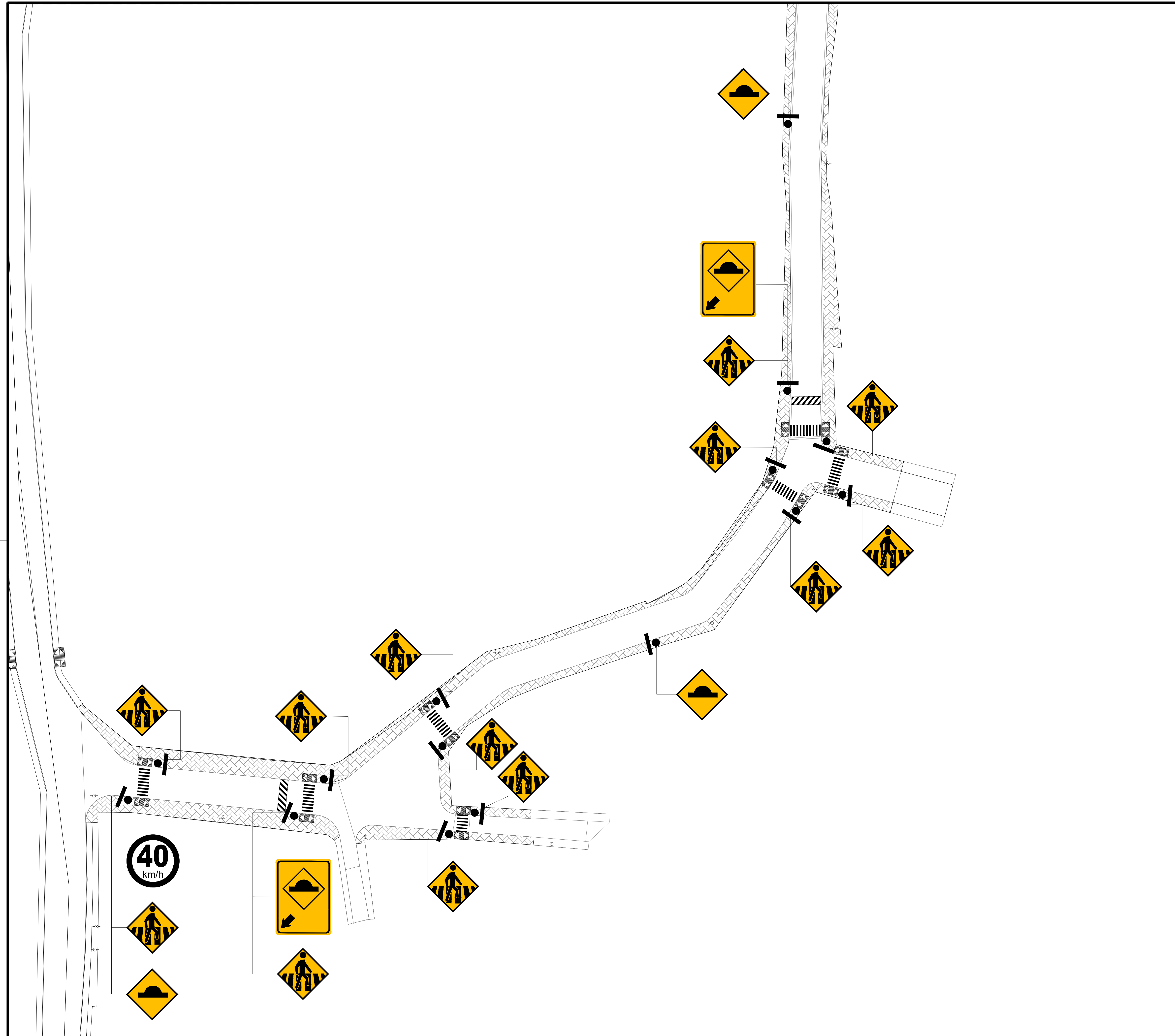
PLANTA BAIXA DE SINALIZAÇÃO ESC:1/350
