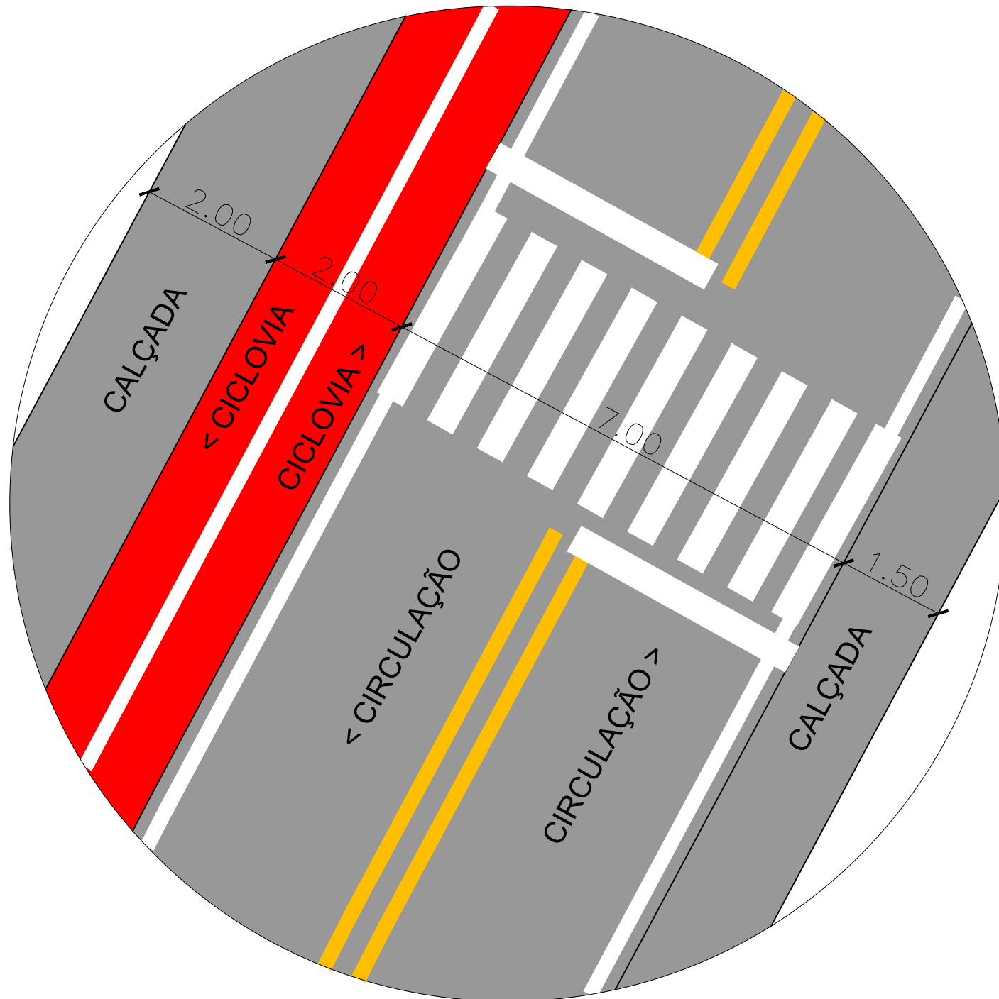
DET. 02 - SEÇÃO DA VIA ESCALA: 1/75
