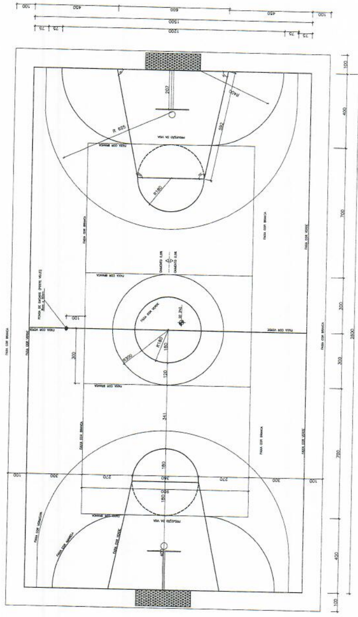
○ PINTURA DO PISO DA QUADRA -- FAIXAS
