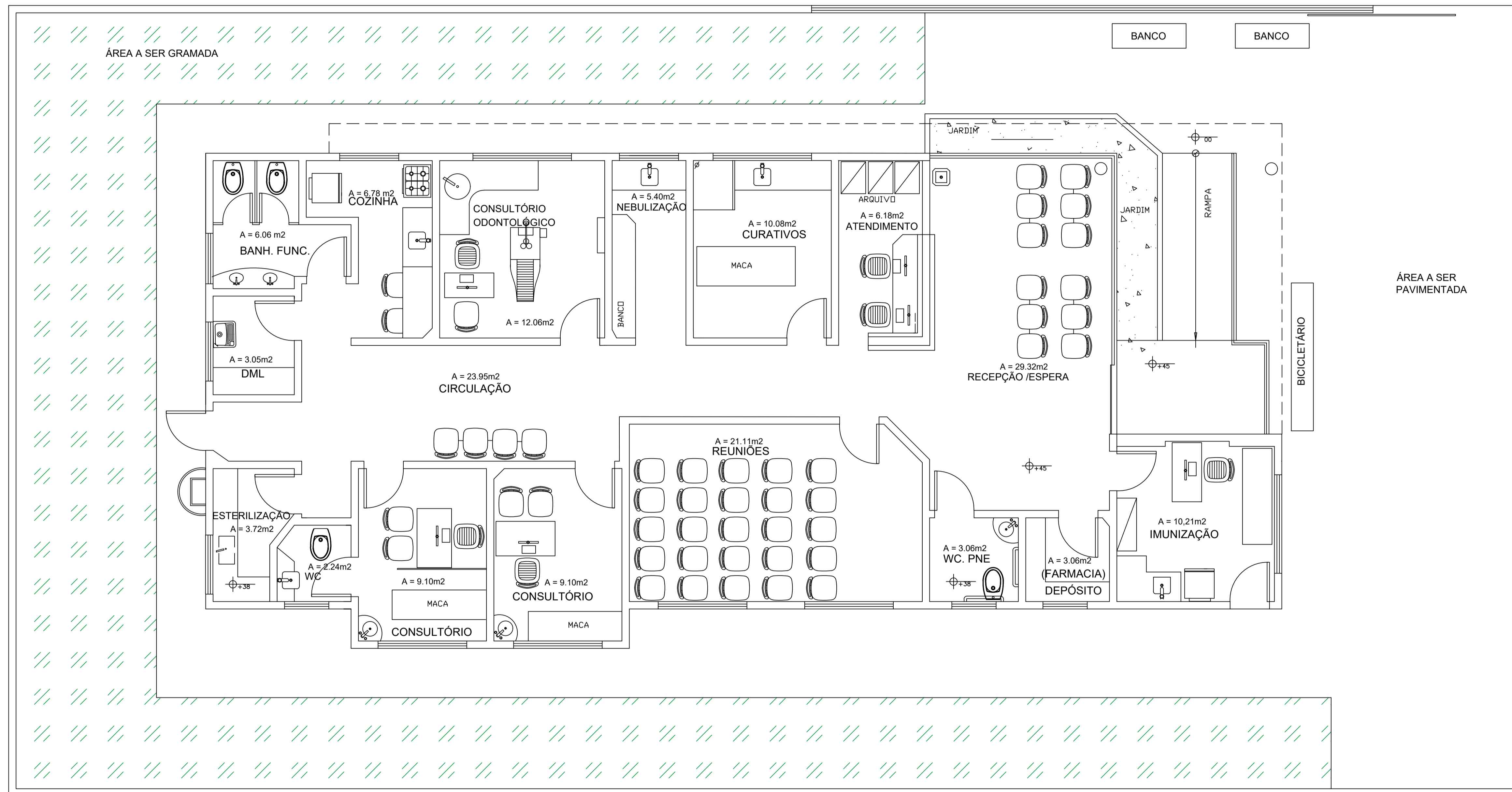
PLANTA DE PAISAGISMO ESC. 1/50
