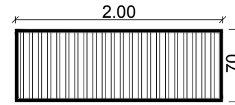
GRADIL - JANELA 03 esc 1:50
