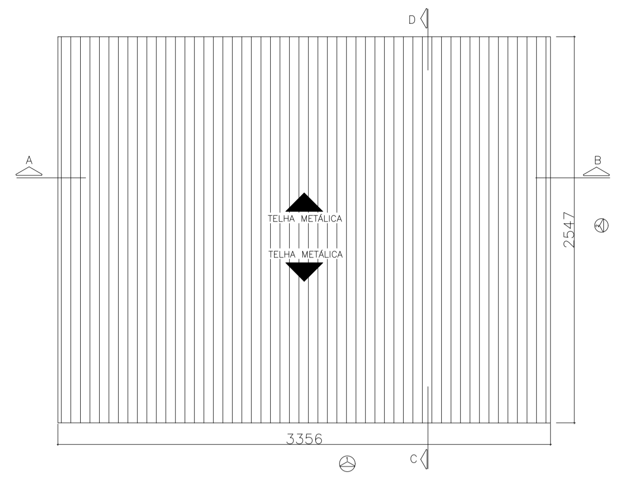
COBERTURA ESQ: 1/250
