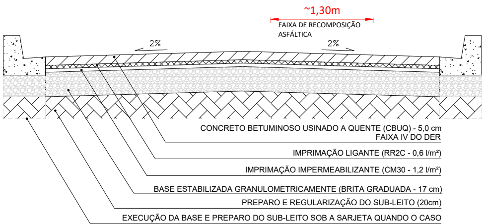
SEÇÃO TIPO DA PAVIMENTAÇÃO SEM ESCALA
