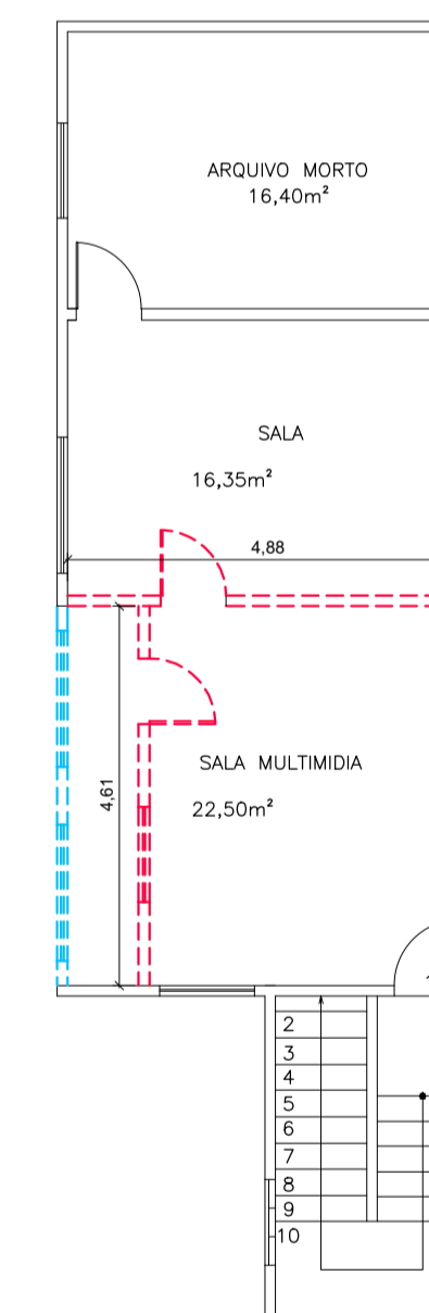
4 PLANTA DE DEMOLIR E CONSTRUIR – 1º PAV. 1/100
