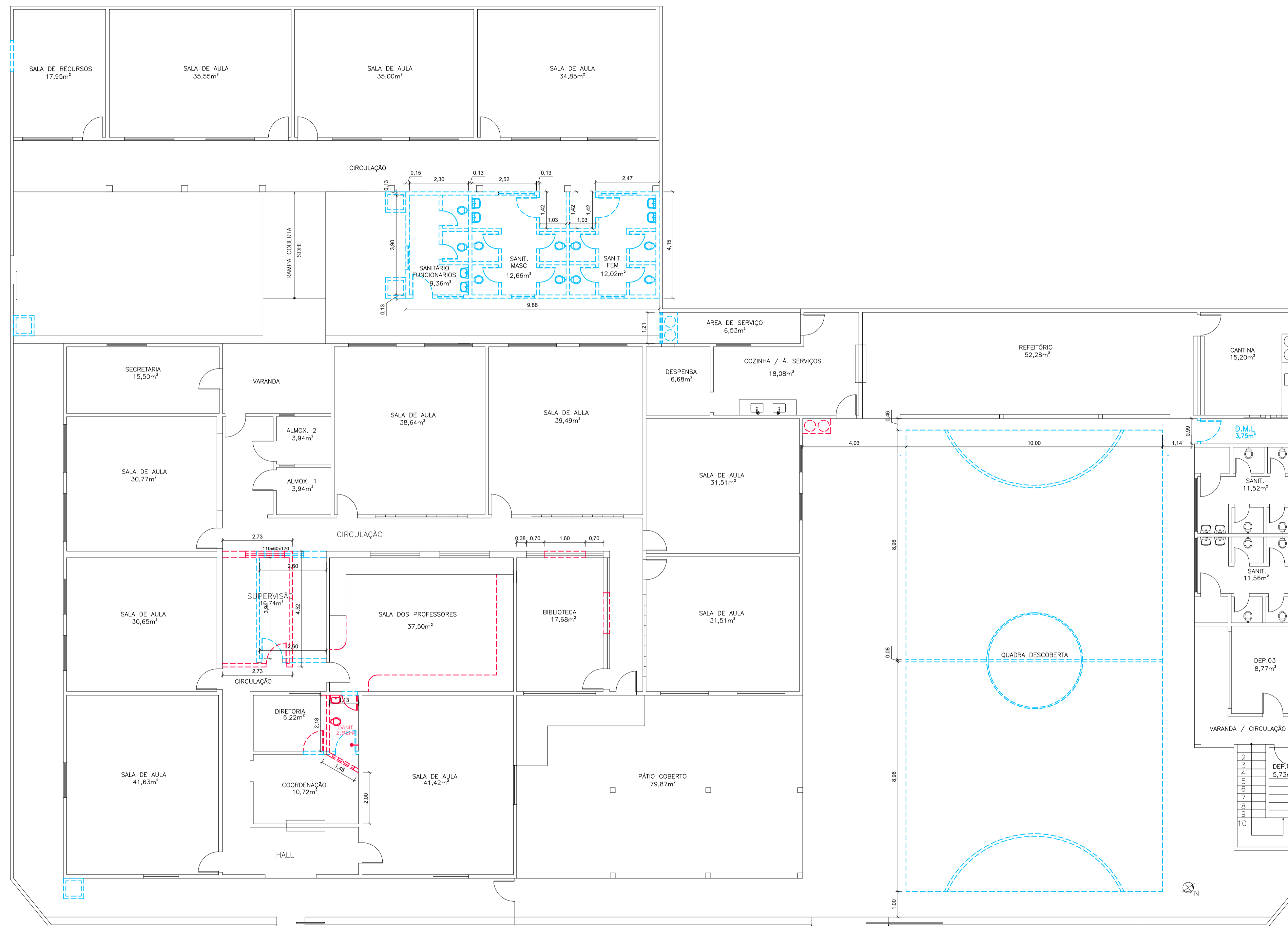
3 PLANTA DE DEMOLIR E CONSTRUIR – TÉRREO 1/100
