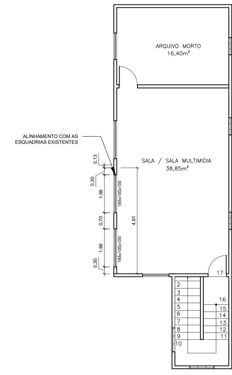
6 PLANTA BAIXA – 1º PAV. 1/100
