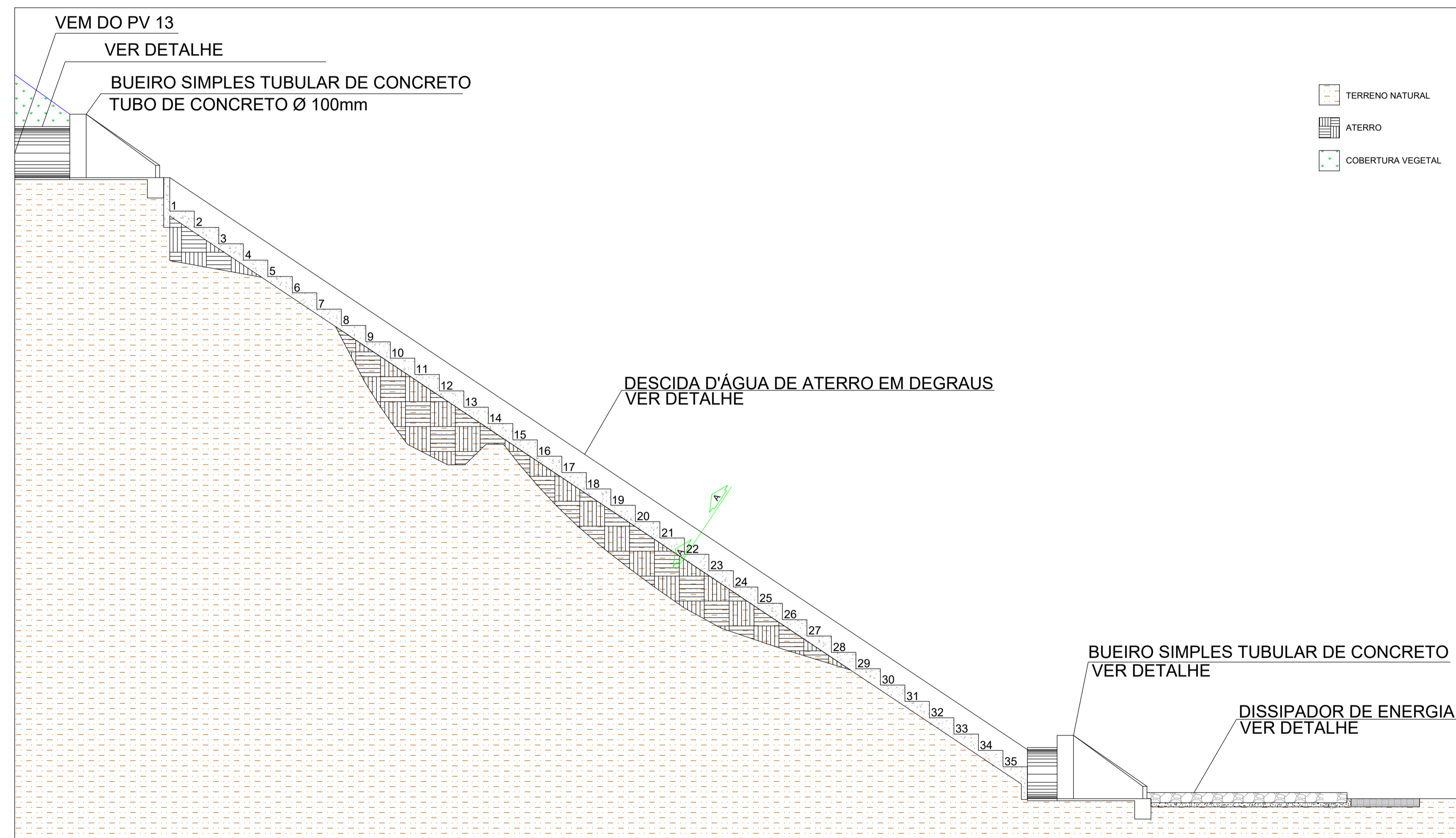
CORTE LONGITUDIANL DESCIDA D'ÁGUA esc 1:75
