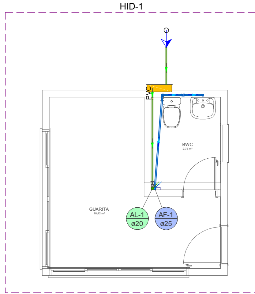
DETALHE HID-1 1:25
