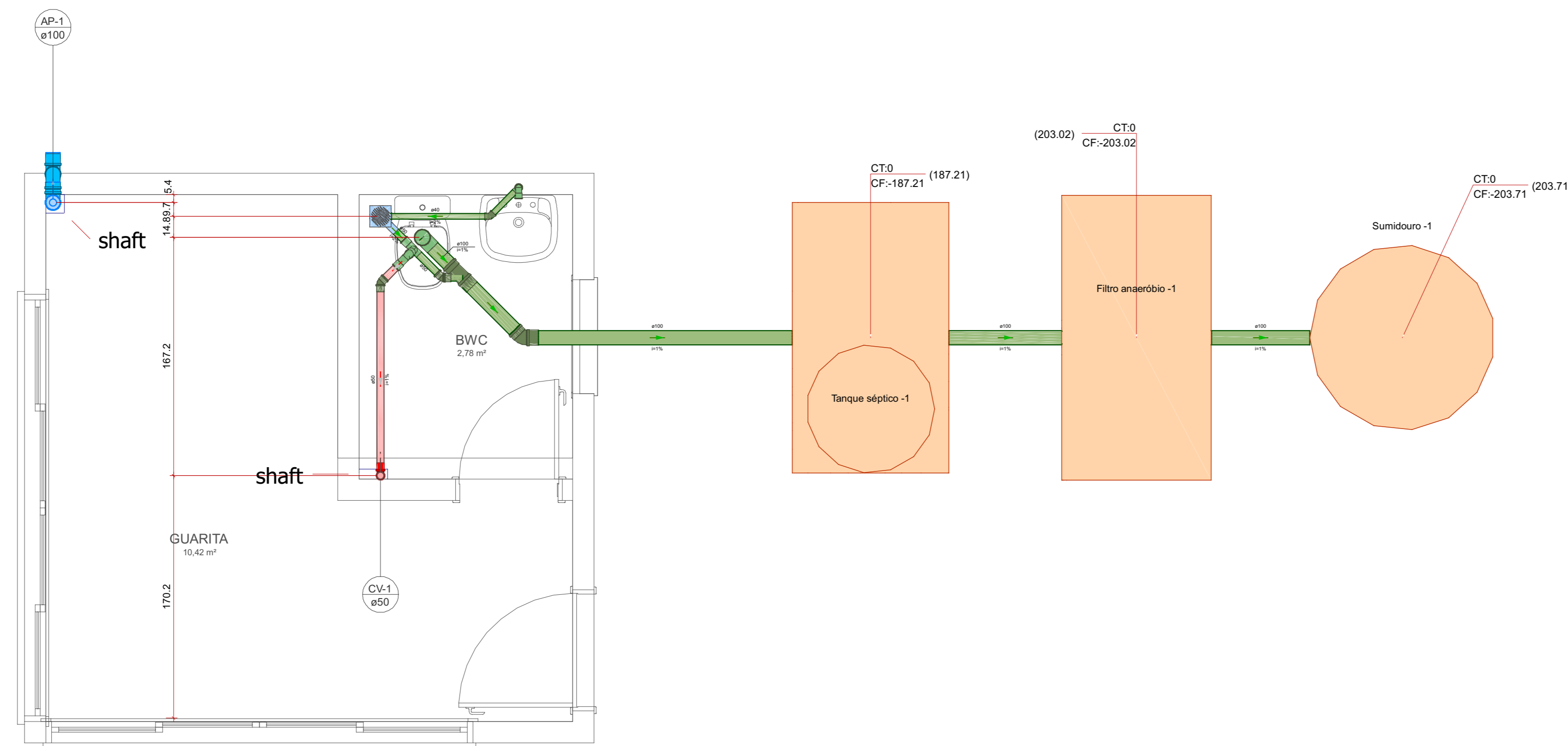
DETALHE SAN-1 1:25
