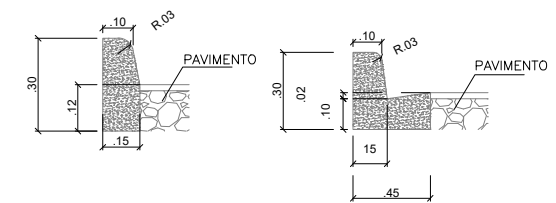
MEIO-FIO (DP-1)
