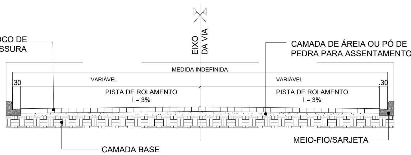
SESSÃO TIPO DA VIA SEM / ESCALA
