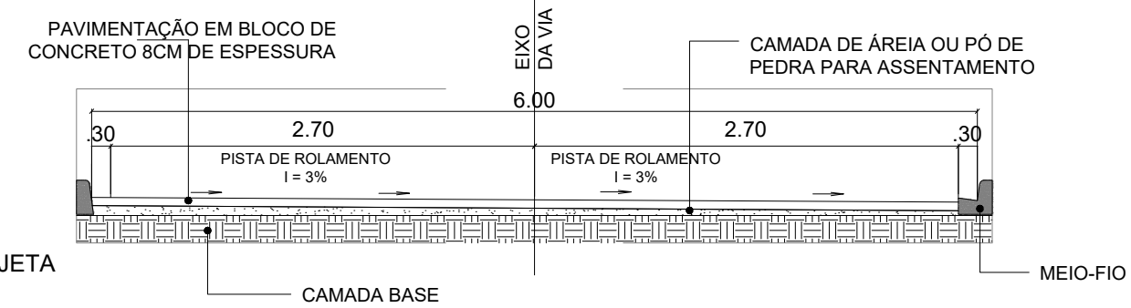
SESSÃO TIPO DA VIA SEM / ESCALA
