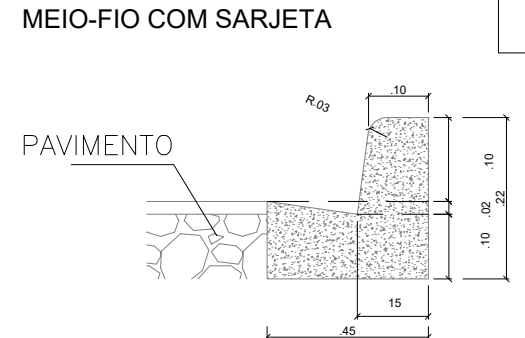
DETALHAMENTO MEIO-FIO E SARJETA SEM / ESCALA
